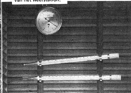
Het instrumentarium van het weerstation.
